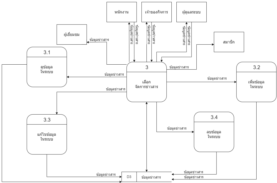
ภาพที่ 3.14 DFD เลือกจัดการข่าวสาร
