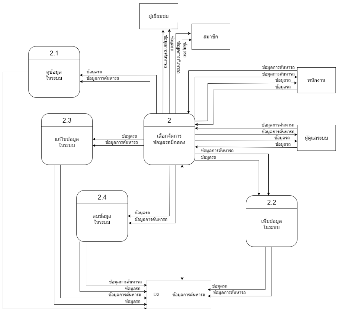
ภาพที่ 3.13 DED เลือกจัดเก็บรถมือสอง
