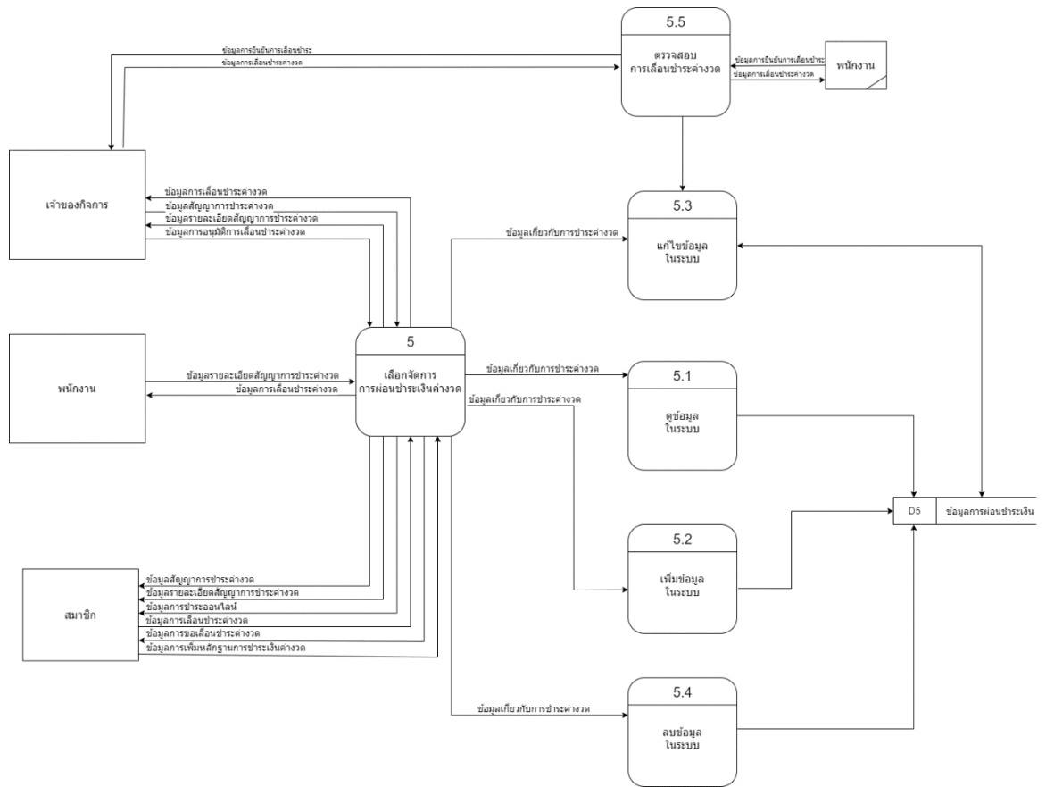
ภาพที่ 3.16 DFD เลือกจัดการการผ่อนชำระเงินค้างงวด
