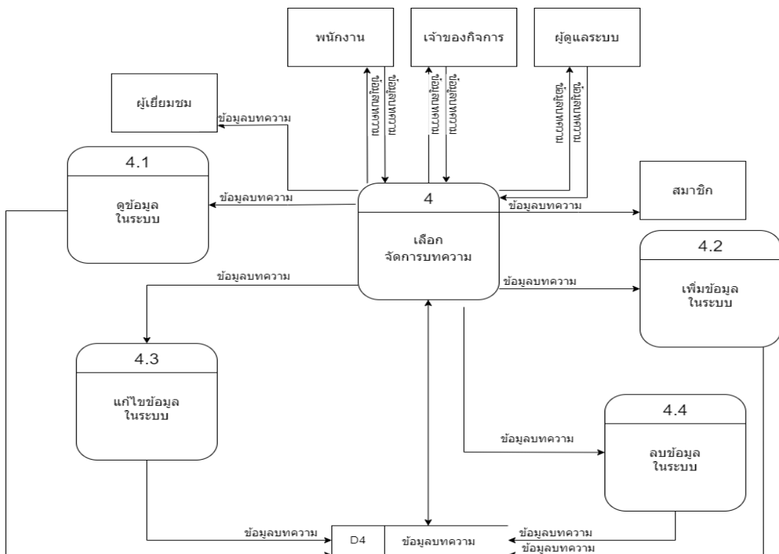
ภาพที่ 3.15 DFD เลือกจัดการบทความ
