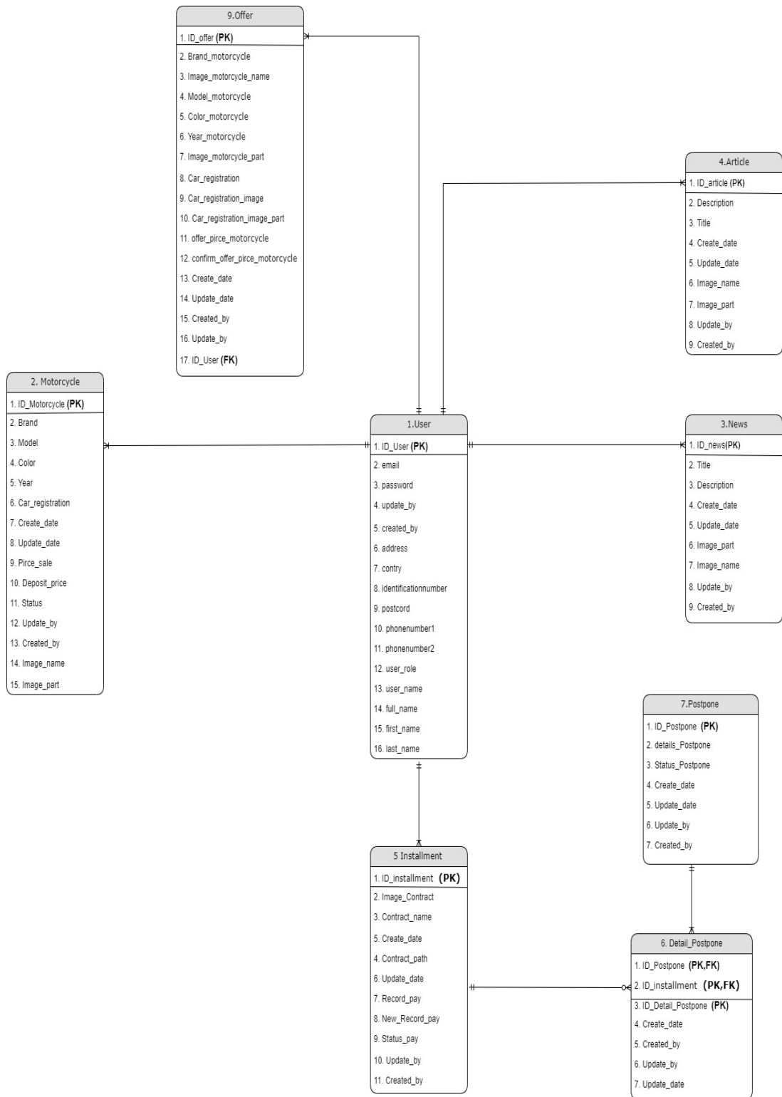
ภาพที่ 3.18 ER- Diagram
