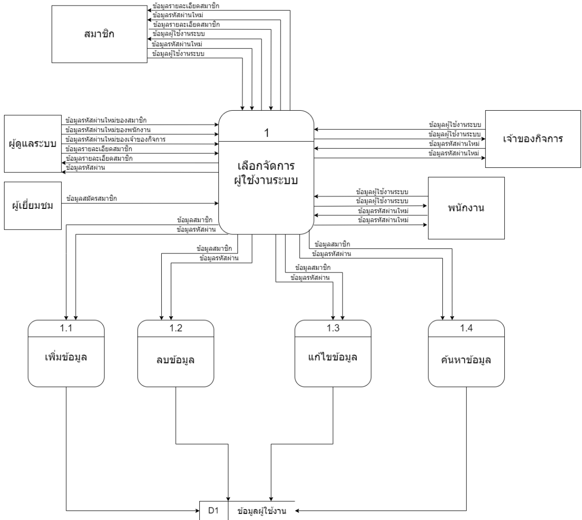
ภาพที่ 3.12 DFD ระบบเลือกจัดการผู้ใช้งานระบบ
